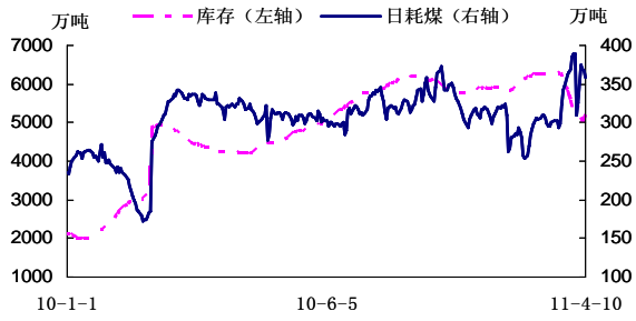
全国重点发电企业存煤、耗煤示意图
